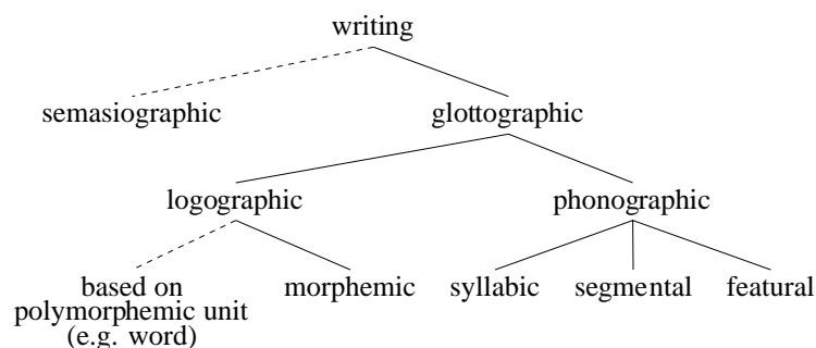
図 1: Sampson の分類
